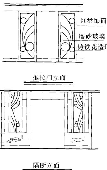
图 6 重点位置装修详图
