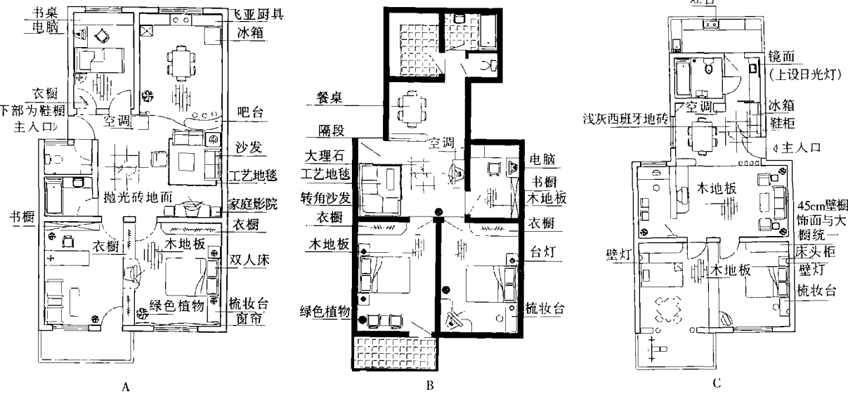
图2 住宅楼中间单元型
